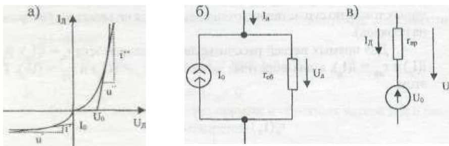
Рис. 1.3. а)-линейная аппроксимация ВАХ;б) - схема замещения по постоянному току обратно смещенного диода; в)- схема замещения диода в прямом включении
